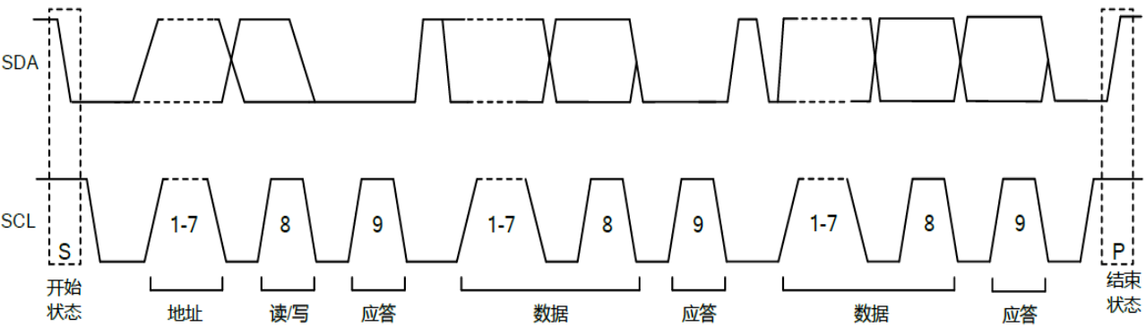
I2C协议
