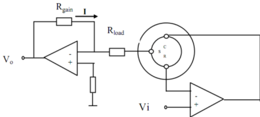
二氧化硫传感器的基本测试电路
