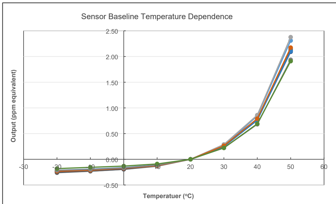
二氧化硫传感器基线的温度依赖性曲线
