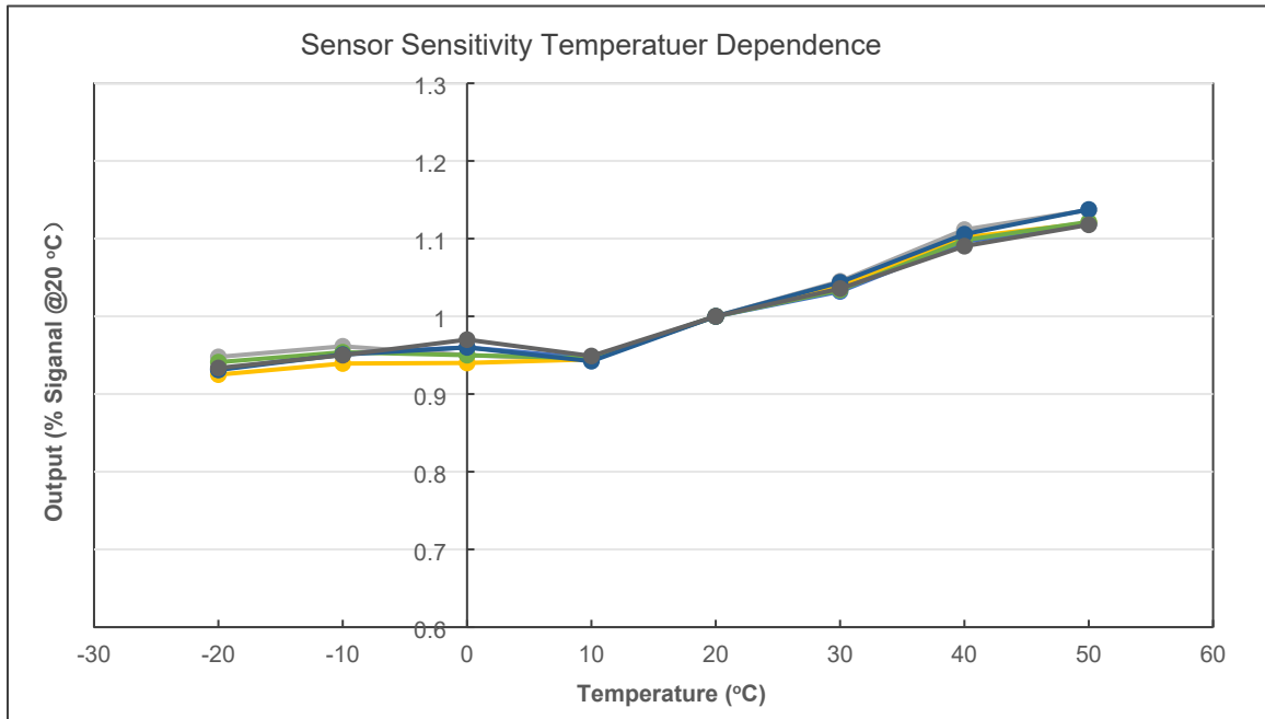
二氧化硫传感器灵敏度的温度依赖性曲线
