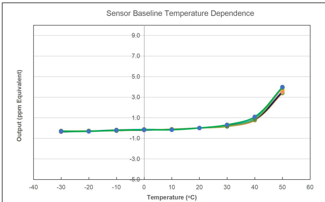
氨气传感器基线的温度依赖性曲线
