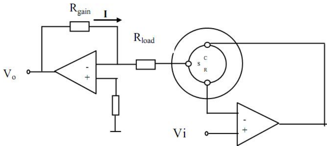
氨气传感器的基本测试电路
