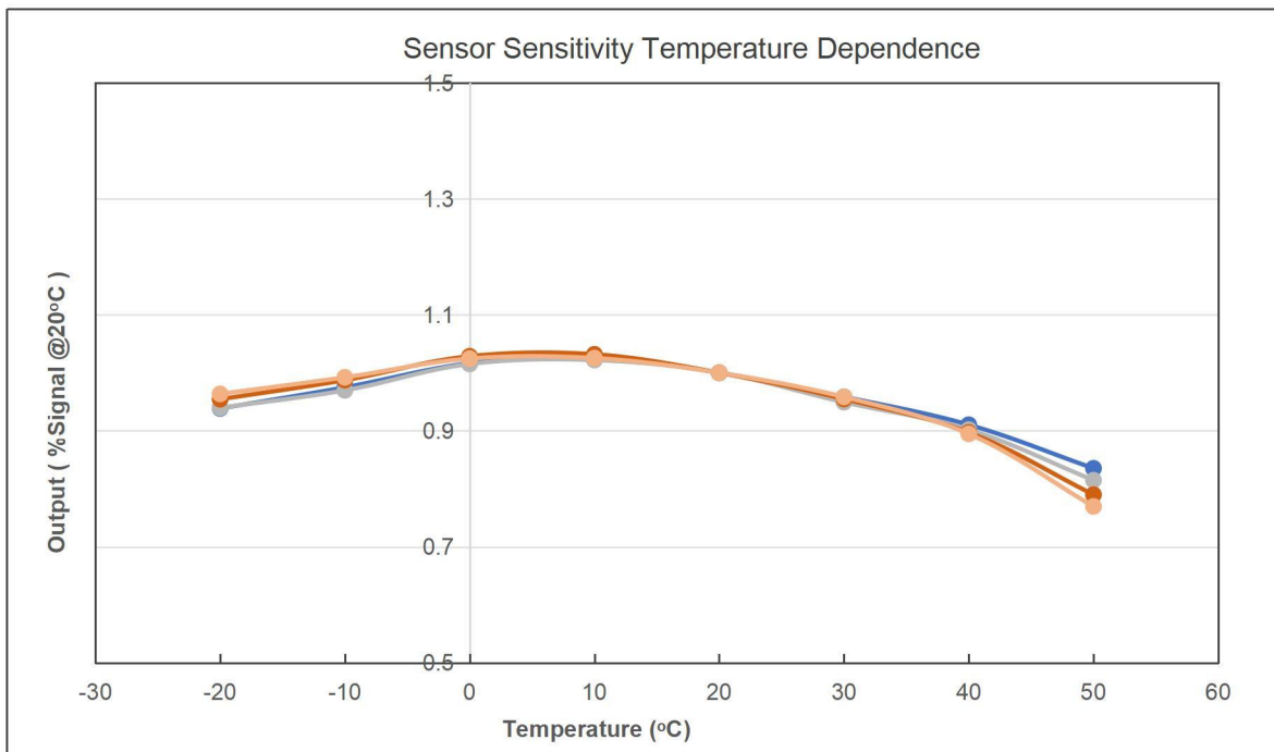
氨气传感器灵敏度的温度依赖性曲线
