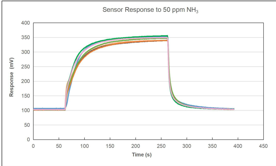
氨气传感器灵敏度的响应恢复曲线
