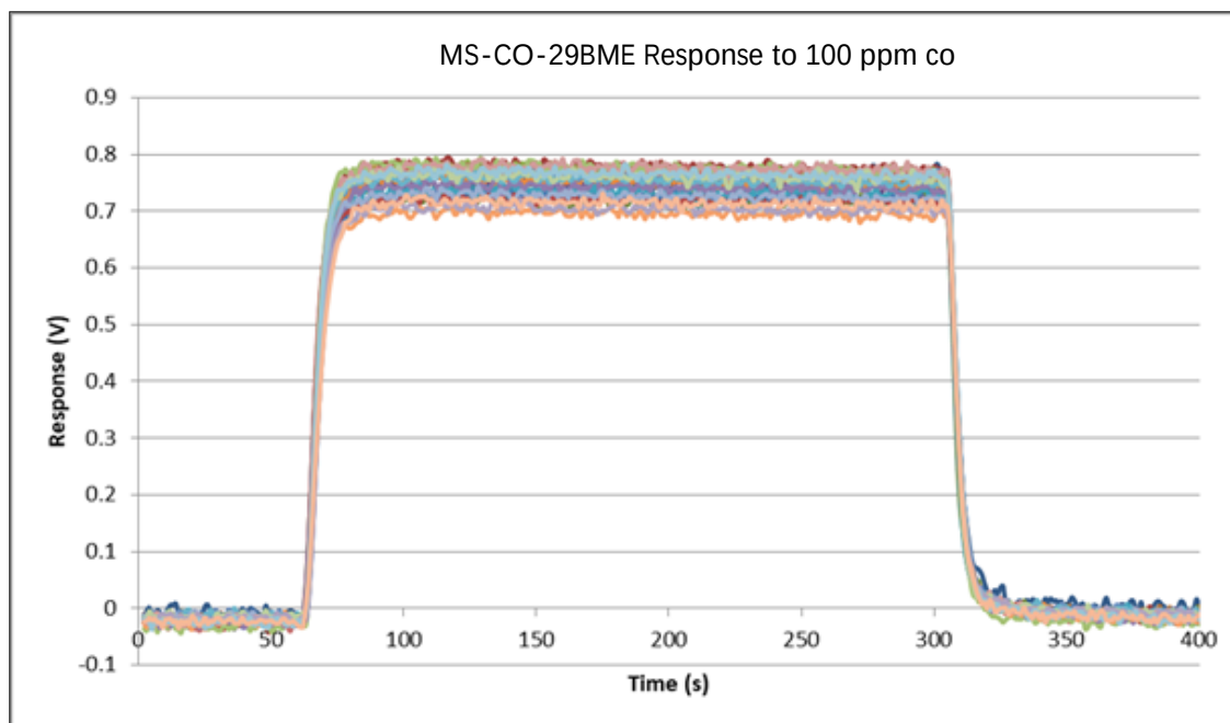
MS-CO-29BME—一氧化碳传感器响应恢复曲线
