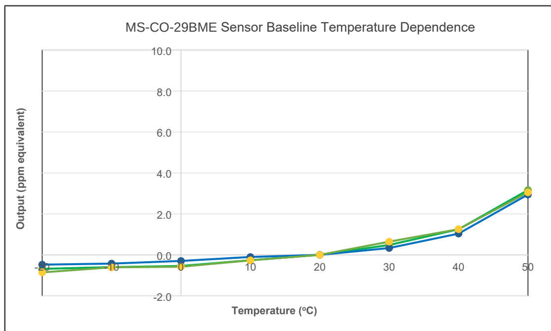
MS-CO-29BME—一氧化碳传感器基线的温度依赖性曲线
