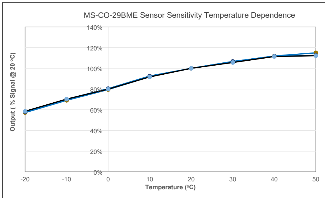
MS-CO-29BME一氧化碳传感器灵敏度的温度依赖性曲线
