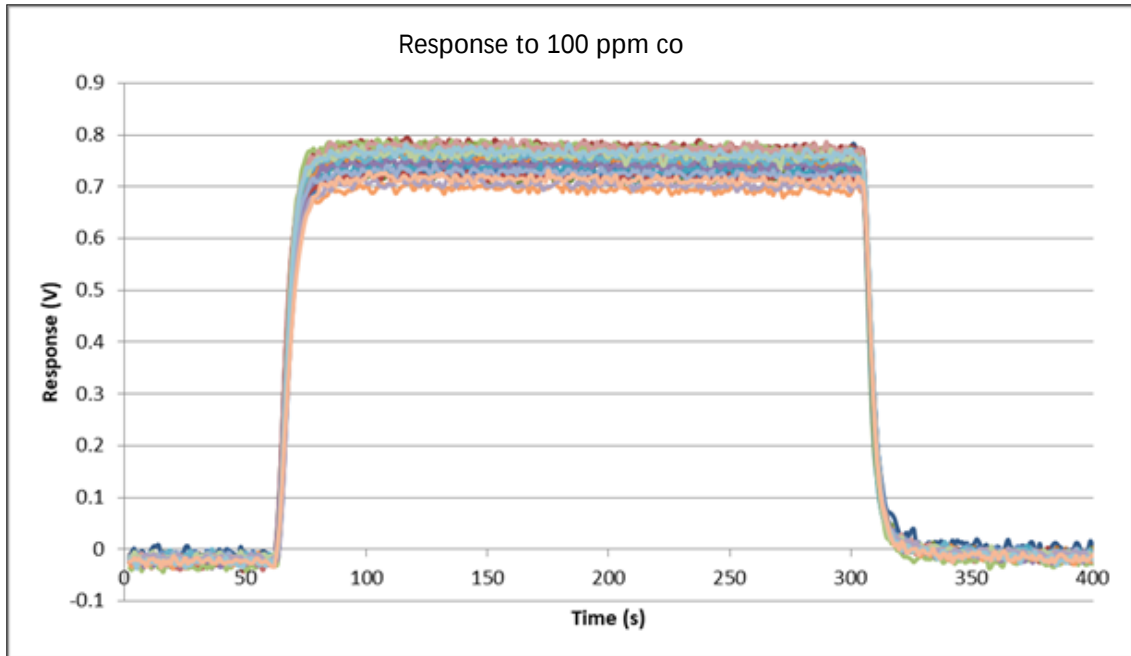
一氧化碳传感器响应恢复曲线
