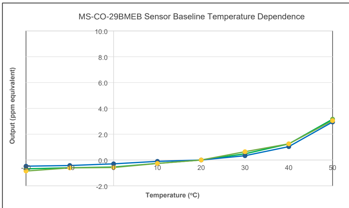
一氧化碳传感器基线的温度依赖性曲线
