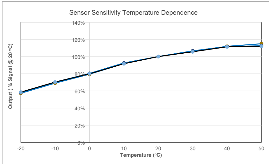
一氧化碳传感器灵敏度的温度依赖性曲线
