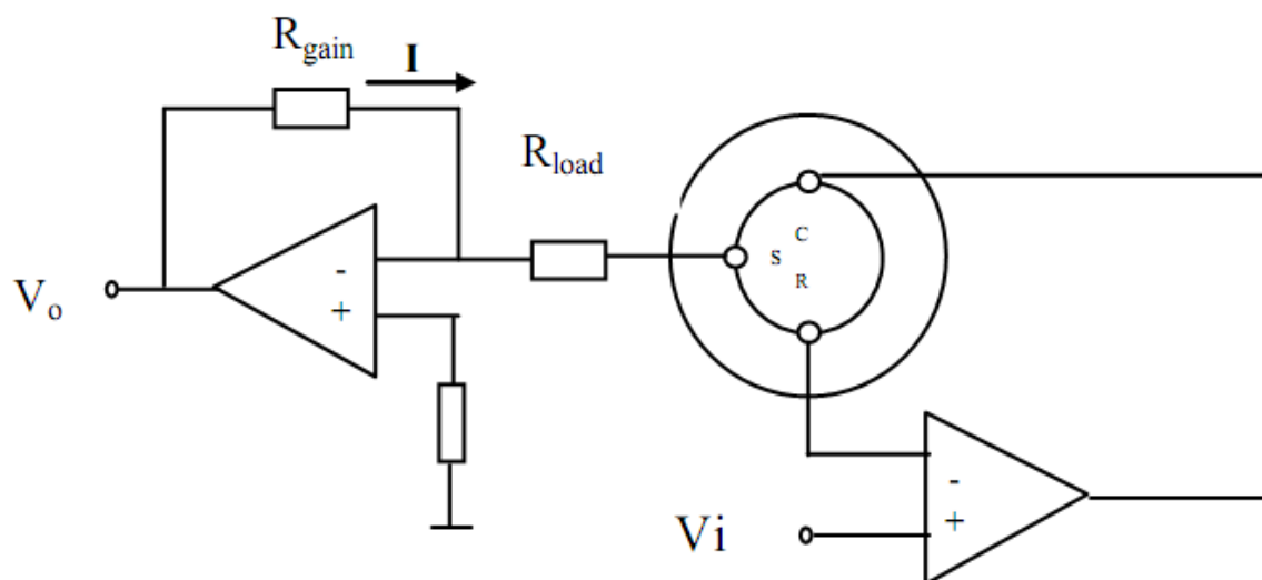
一氧化碳传感器的基本测试电路
