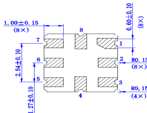
底视尺寸图(单位: mm)
