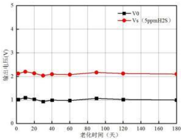
图 7 长期稳定特性曲线
