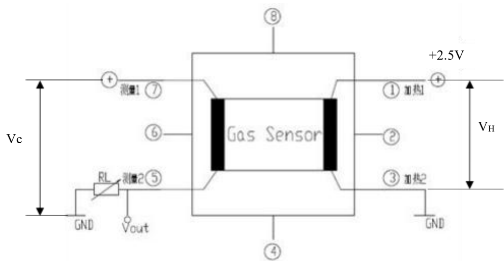
图 2 测试电路
