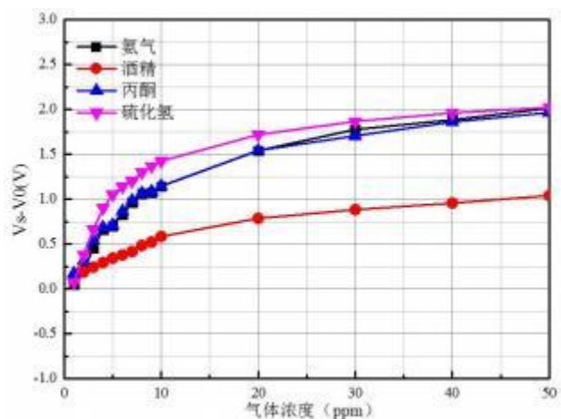
图 6 传感器线性特性曲线
