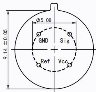
底视图
