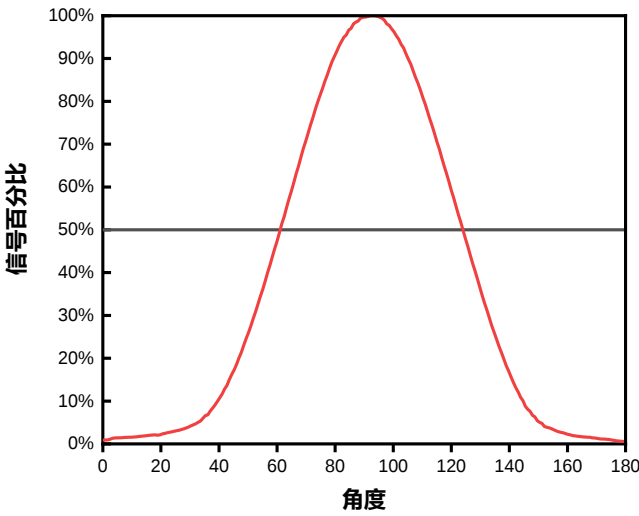
MS-TP-36BPDG视场角
