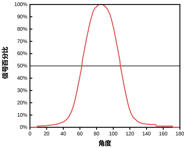
MS-TP-36BPDG-A视场角
