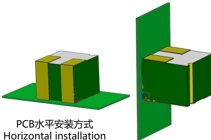
PCB垂直安装方式 Vertical installation
