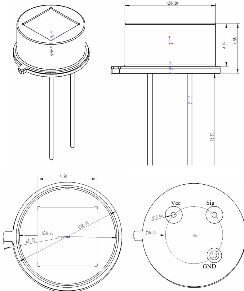
探测器封装尺寸图
