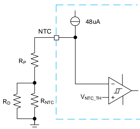
Fig. 5. NTC Protection
