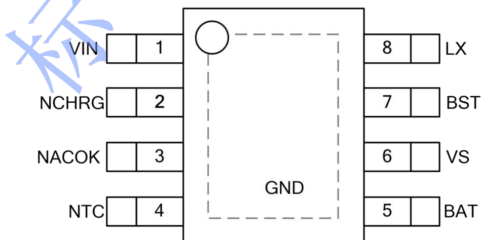
图 4 引脚封装图
