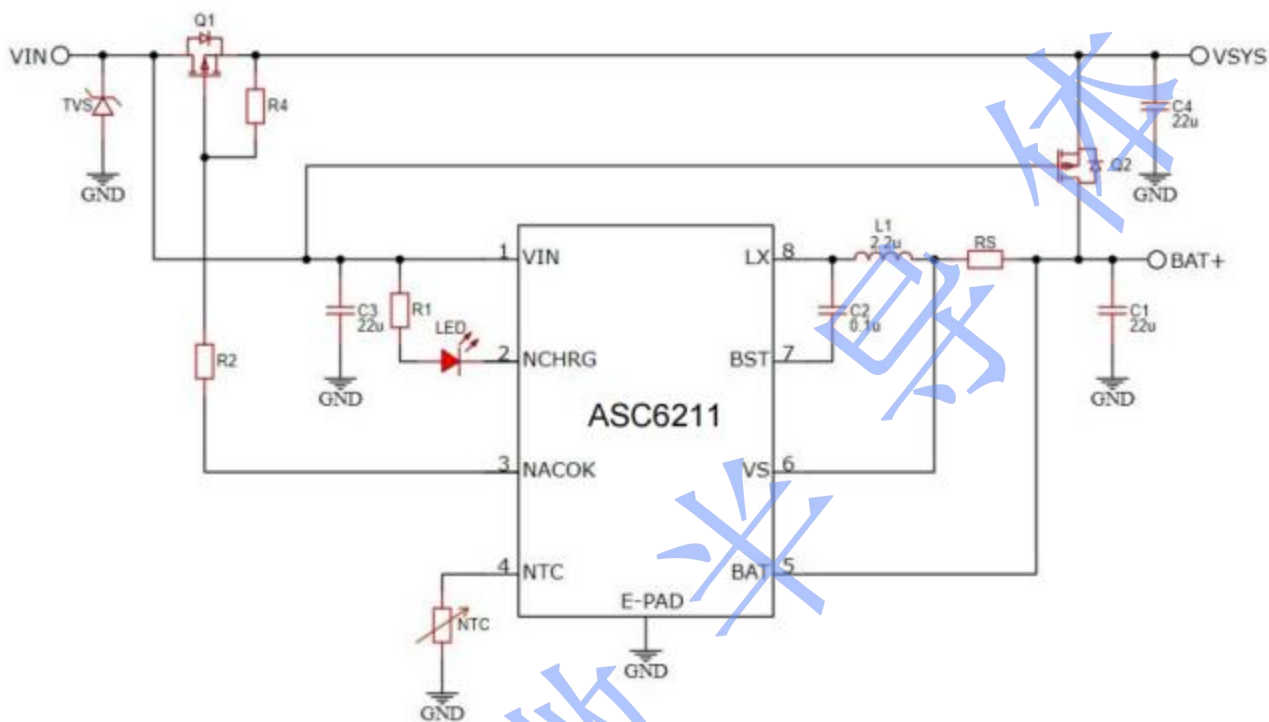
图 6 带路径管理的扩展应用
